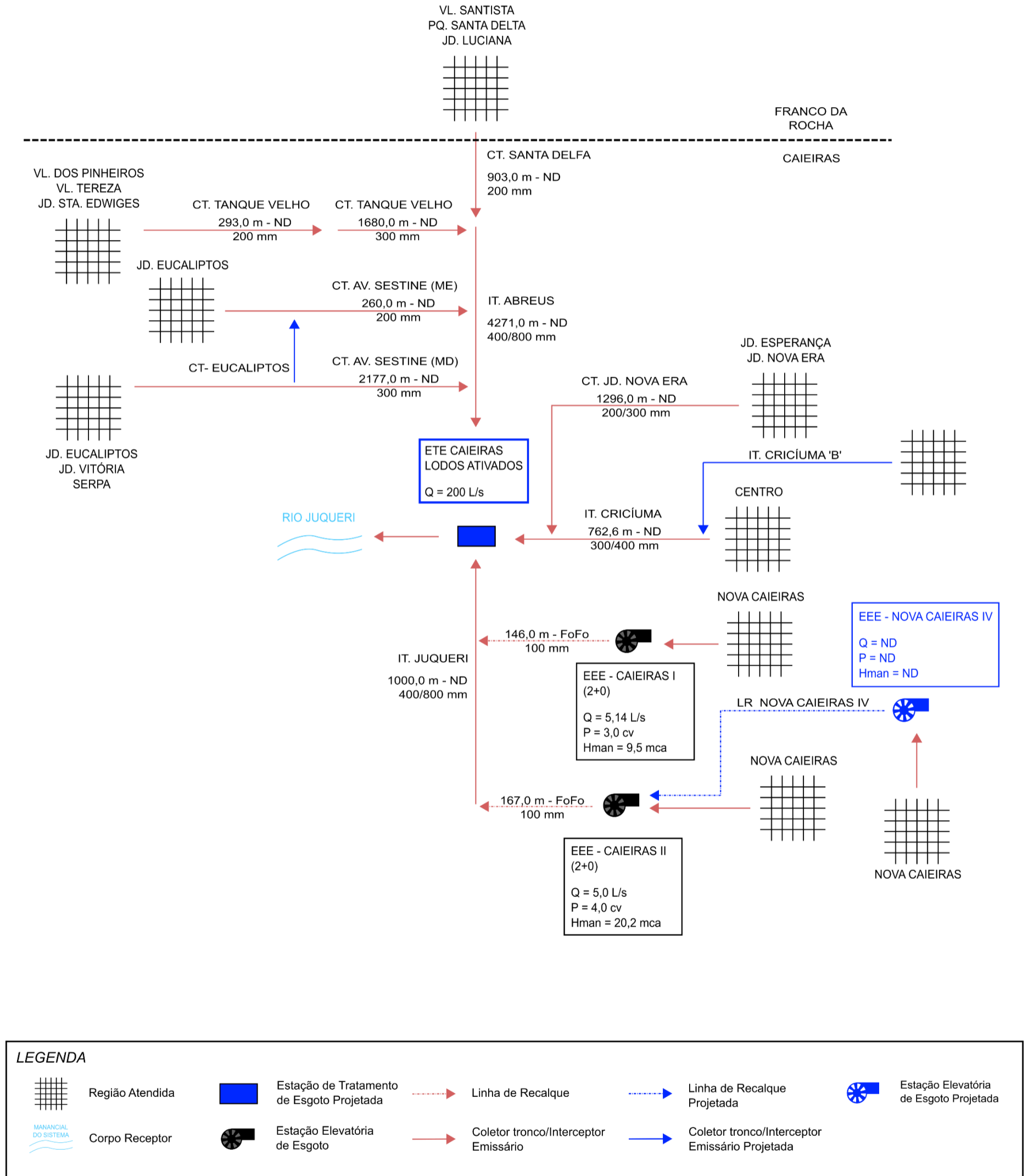
Figura 4.4 – Croqui do Sistema de Esgotamento Sanitário de Caieiras e Franco da Rocha – ETE Caieiras.
